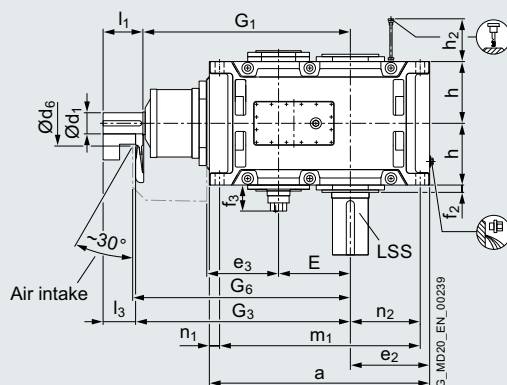
B2.V Dip lubrication 2LP302-...02-....
