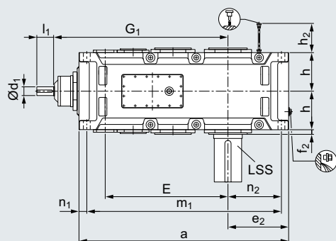
B4.V Dip lubrication 2LP302-...22-....
