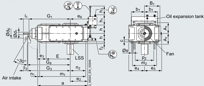
B3.V Dip lubrication 2LP302-...12-....
